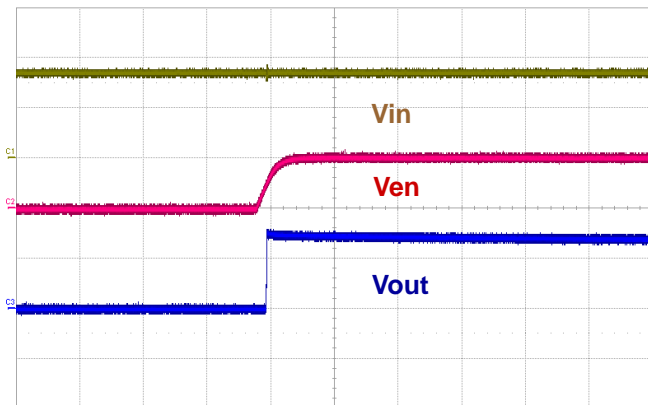
VIN : 2.0V/div, VEN : 2.0V, VOUT : 2.0V/div, Time : 1m/div
