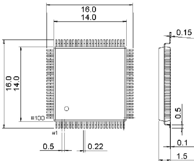
图 5-5 LQFP100 封装
