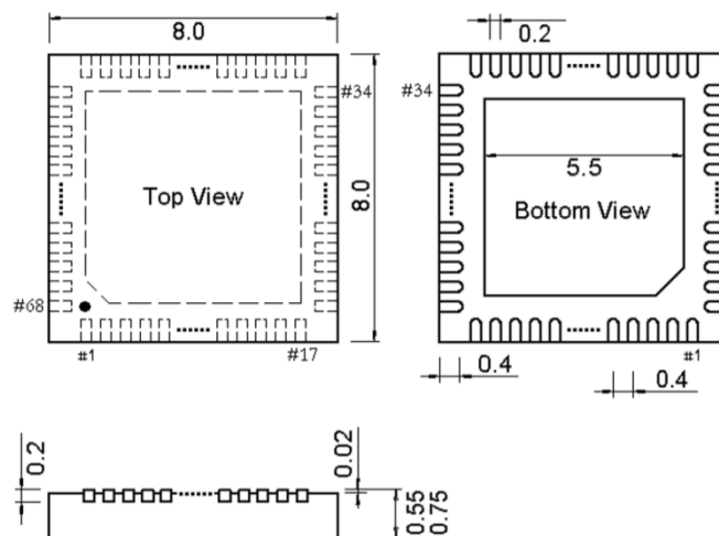
图 5-2 QFN68X8 封装
