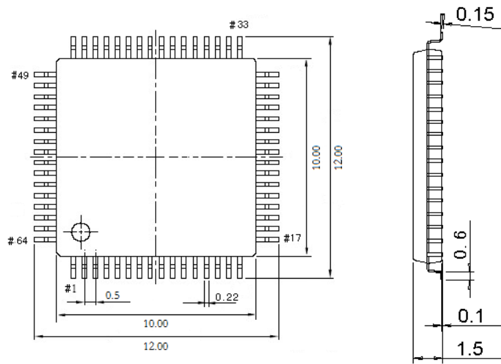
图 5-4 LQFP64M 封装
