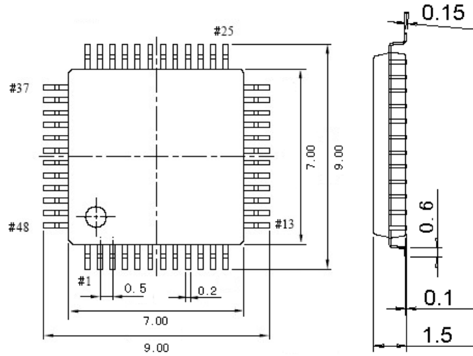
图 5-3 LQFP48 封装
