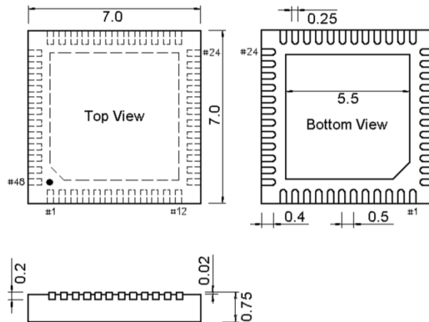
图 5-1 QFN48X7 封装
