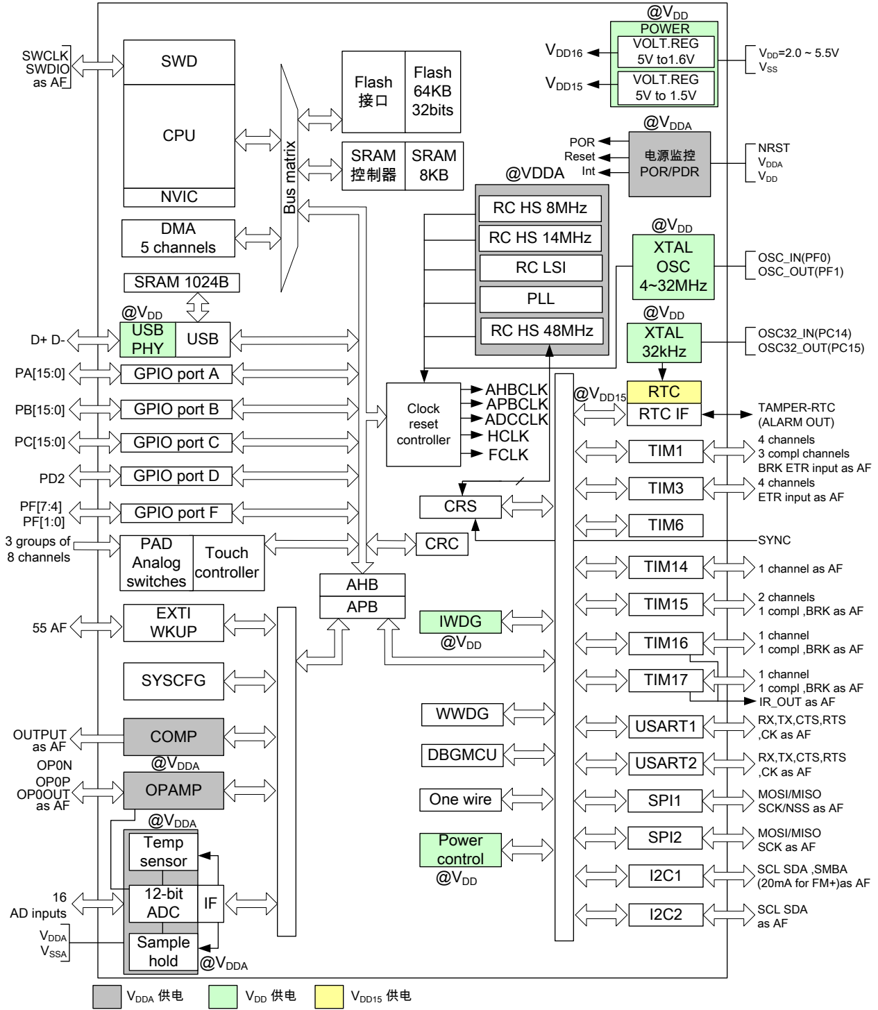
图 2.1 系统框图
