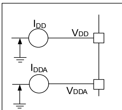
图 6.4 电流消耗测量方案
