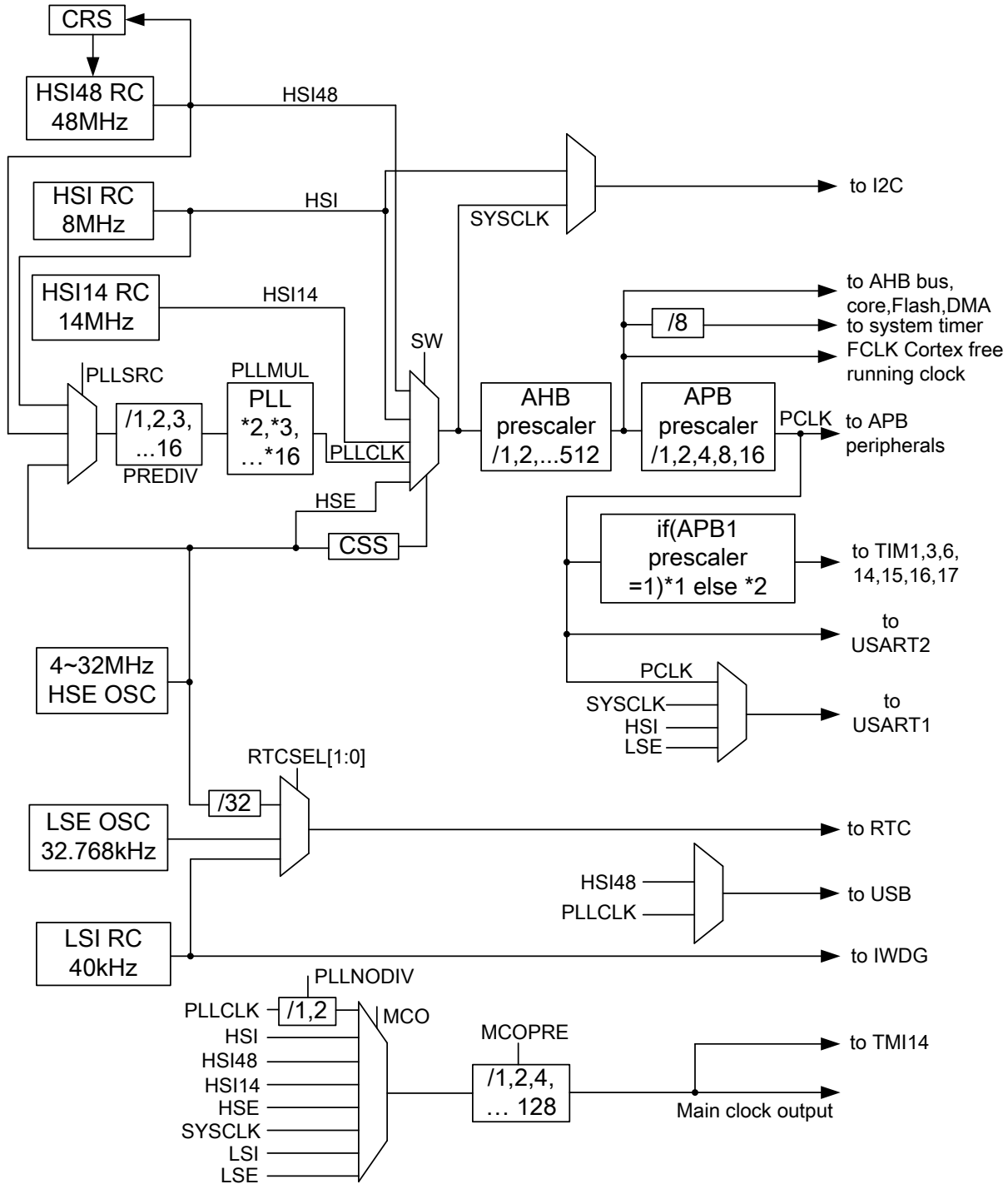
图 3.1 时钟框图
