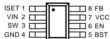
APW7315 TSOT-23-8A
