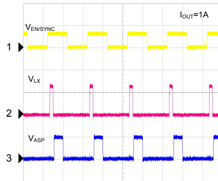
ASP Output
