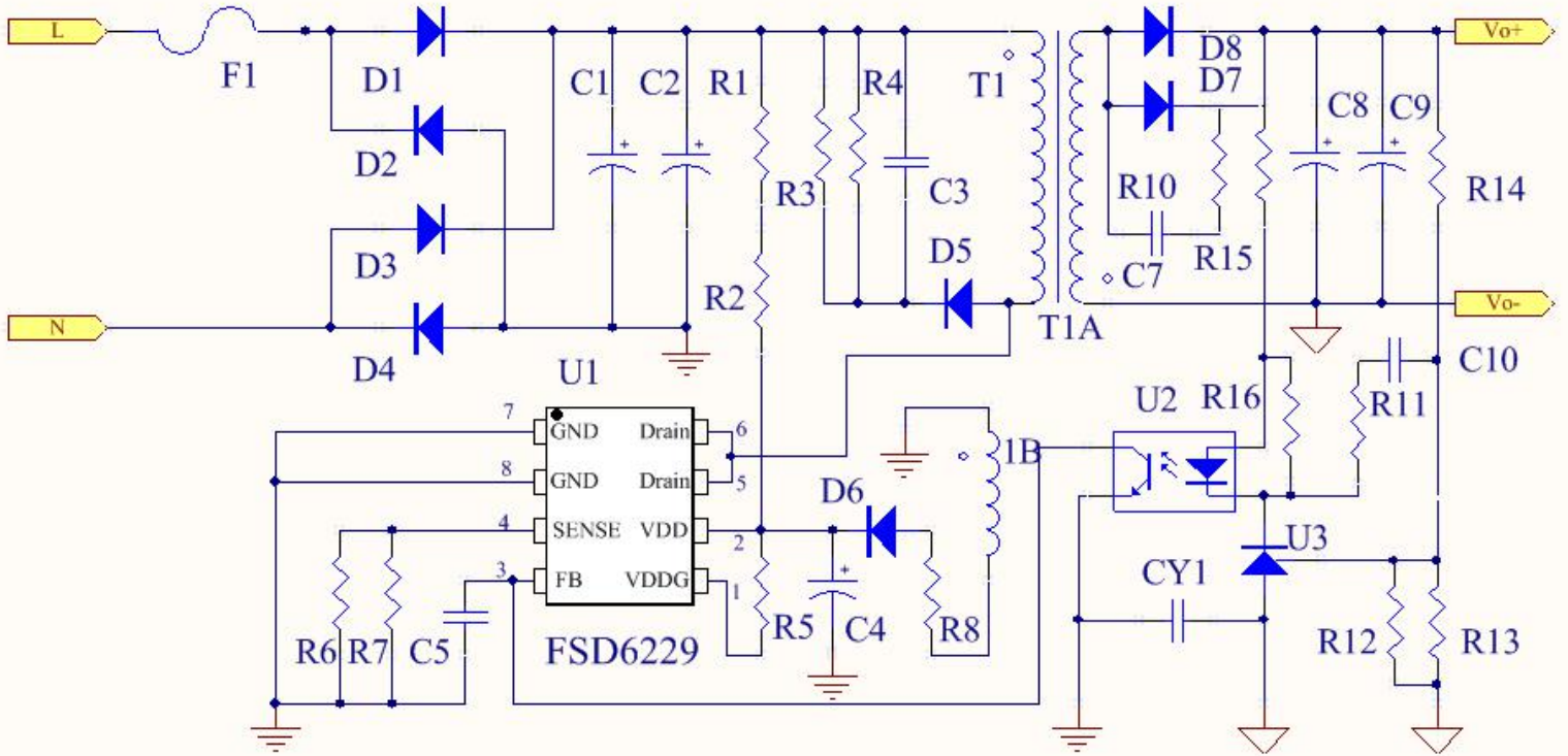
图 2.典型应用图
