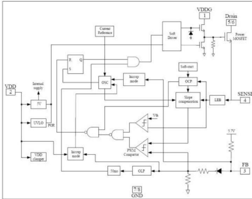
图1. 电路功能框图
