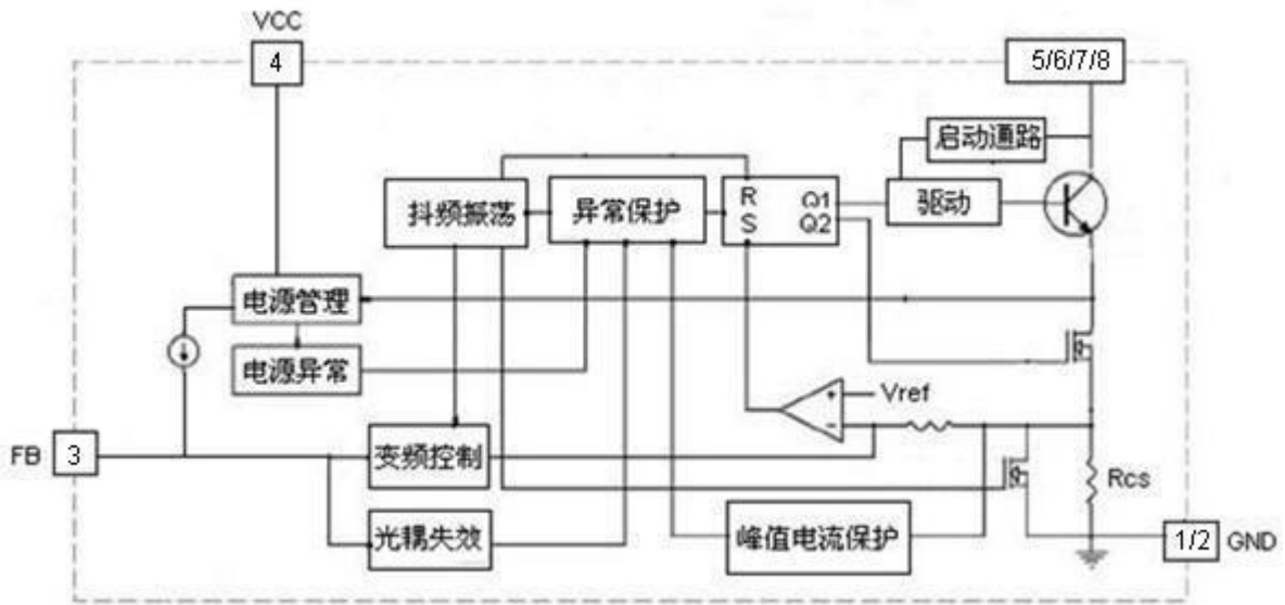
图1. 电路功能框图
