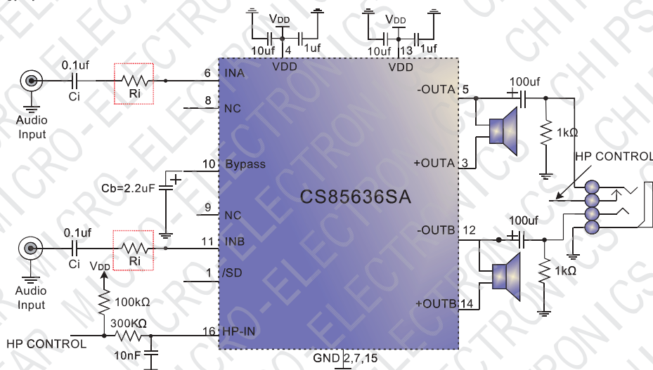
图 1 CS85636SA应用线路图
