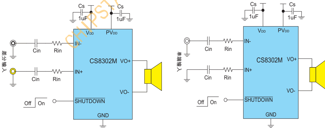
图2 CS8302单端输入方式应用图
