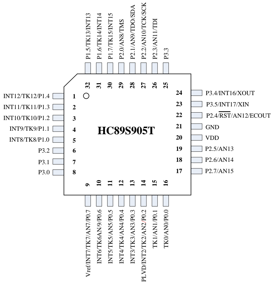
Figure 1-1 LQFP32 引脚配置图
