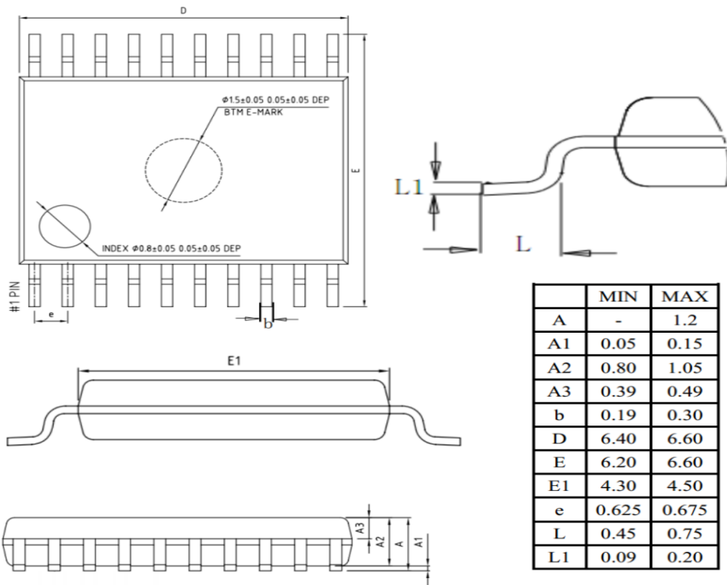
Figure 26-2 TSSOP20 封装尺寸
