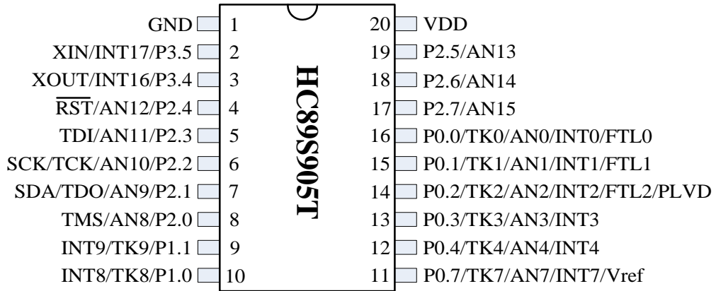
Figure 1-2 TSSOP20 引脚配置图
